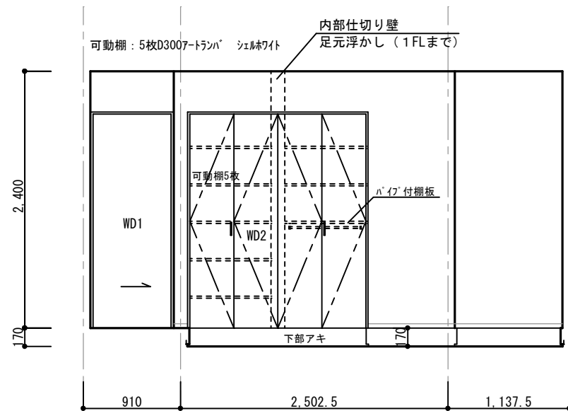
玄関 東面
