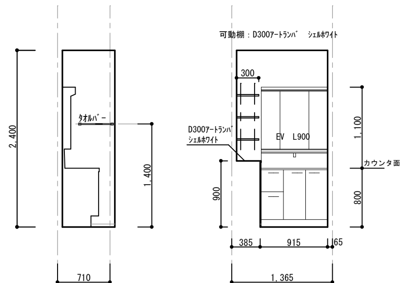
1階洗面 西面
