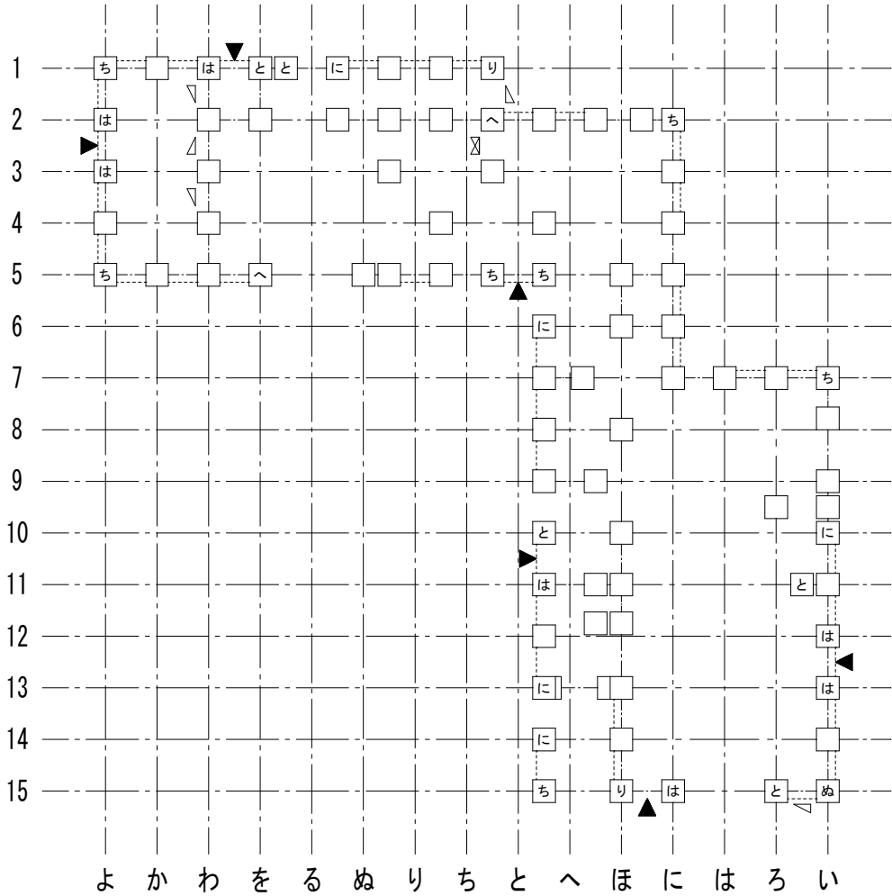
1 階柱壁伏図
