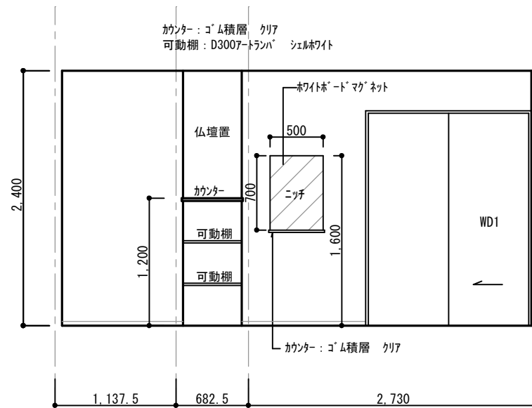
LDK 西面
