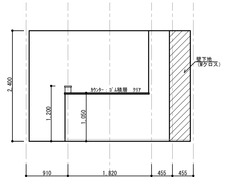
LDK 北面
