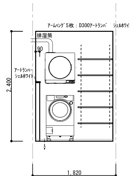
脱衣室 東面
