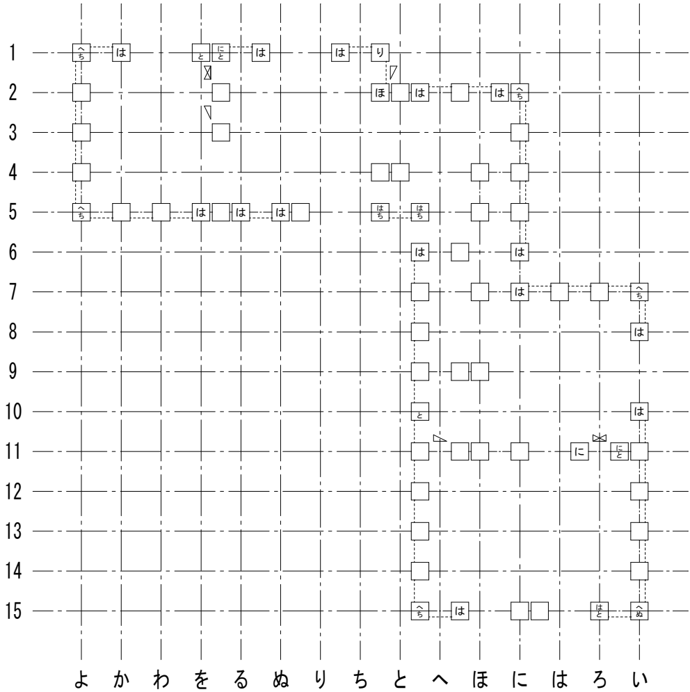
2 階柱壁伏図
